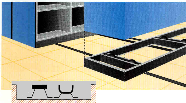
Raíles para empotrar en el pavimento.
