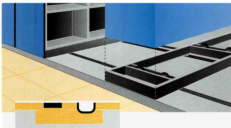
Raíles en plataforma de madera reforzada sin necesidad de obras.
